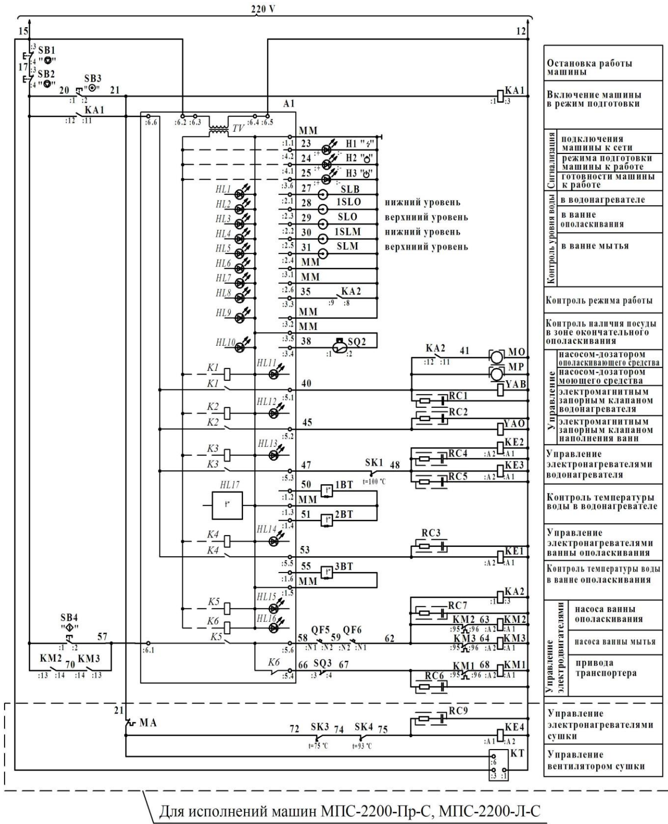
Рисунок 3 (лист 2 из 2) – Схема электрическая принципиальная
